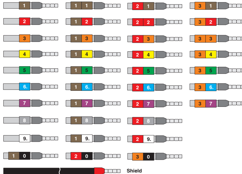
Rysunek schematyczny
