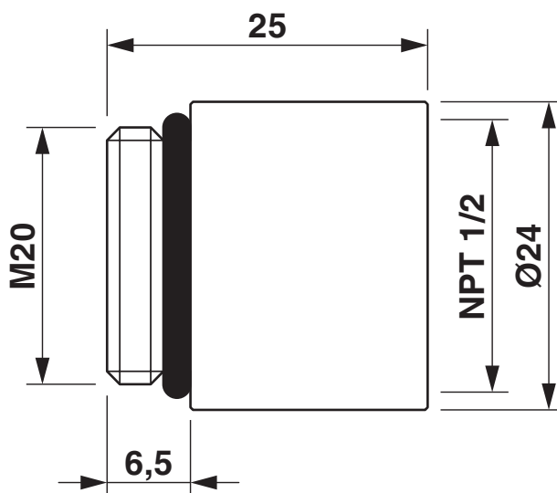
Rysunek wymiarowy
