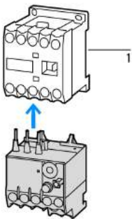
1 styczniki mocy
