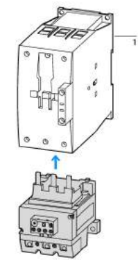
1 Stycznik mocy 2 cokół
