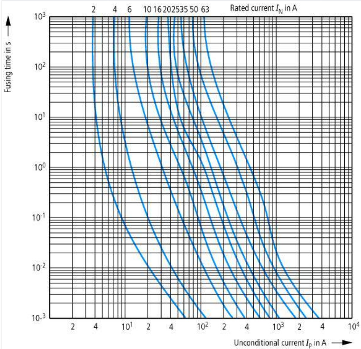
Charakterystyka czasowo-prądowa wkładki topikowej D0 2...63 A gG(gL)
