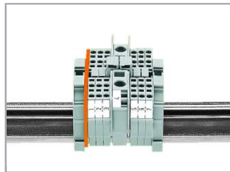
Mostkowanie redukcyjne złączek listwowych 6 mm 2 (seria 282) ze złączkami listwowymi 1,5 mm 2 (seria 279)
