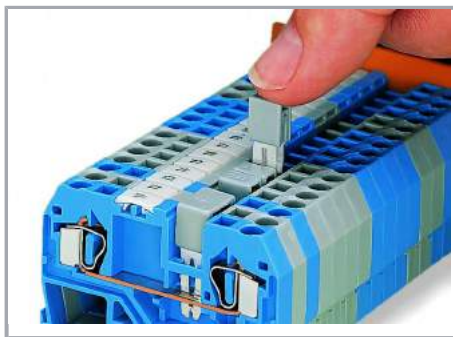
Mostkowanie przy pomocy mostka poprzecznego (280-402)
