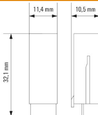
Rysunek wymiarowany
