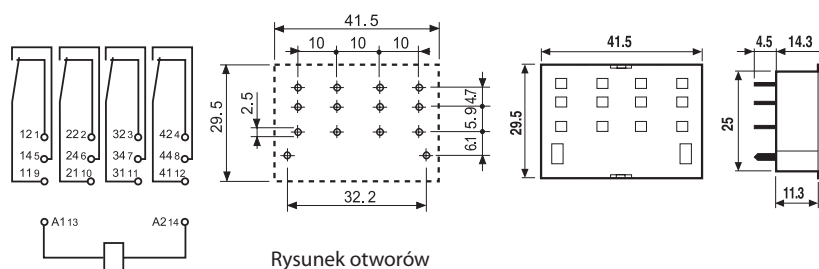
Rysunek otworów montażowych 96.12
