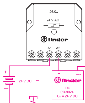
Schemat łączy dla sterowania wyłącznikiem impulsowego, seria 26 zasilanie 24 V DC.
