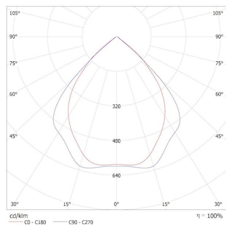
KANLUX S.A. (kat 38491) ACETE 20W CCT GR / Krzywa rozsyłu światła (biegunowo)
