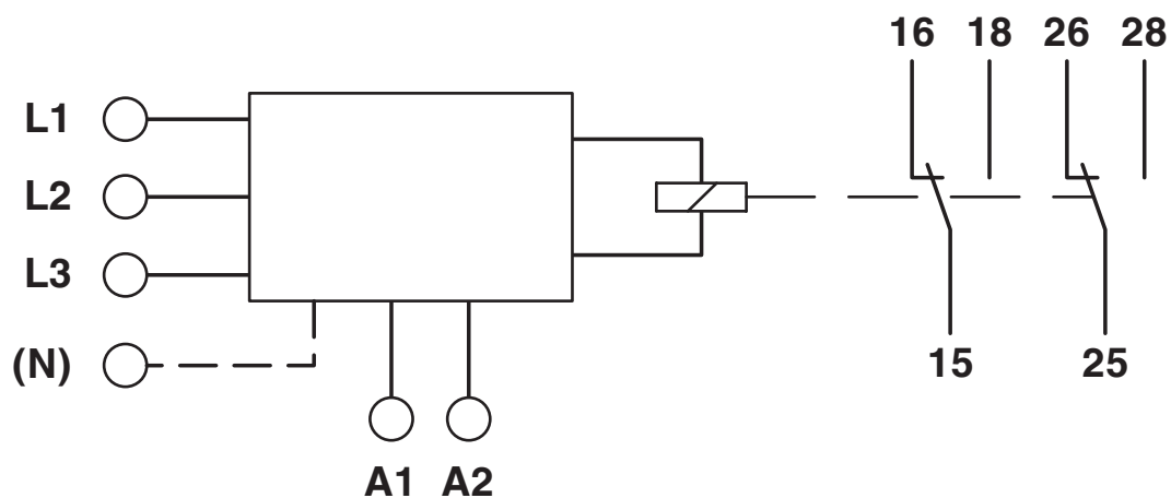
Schemat blokowy
