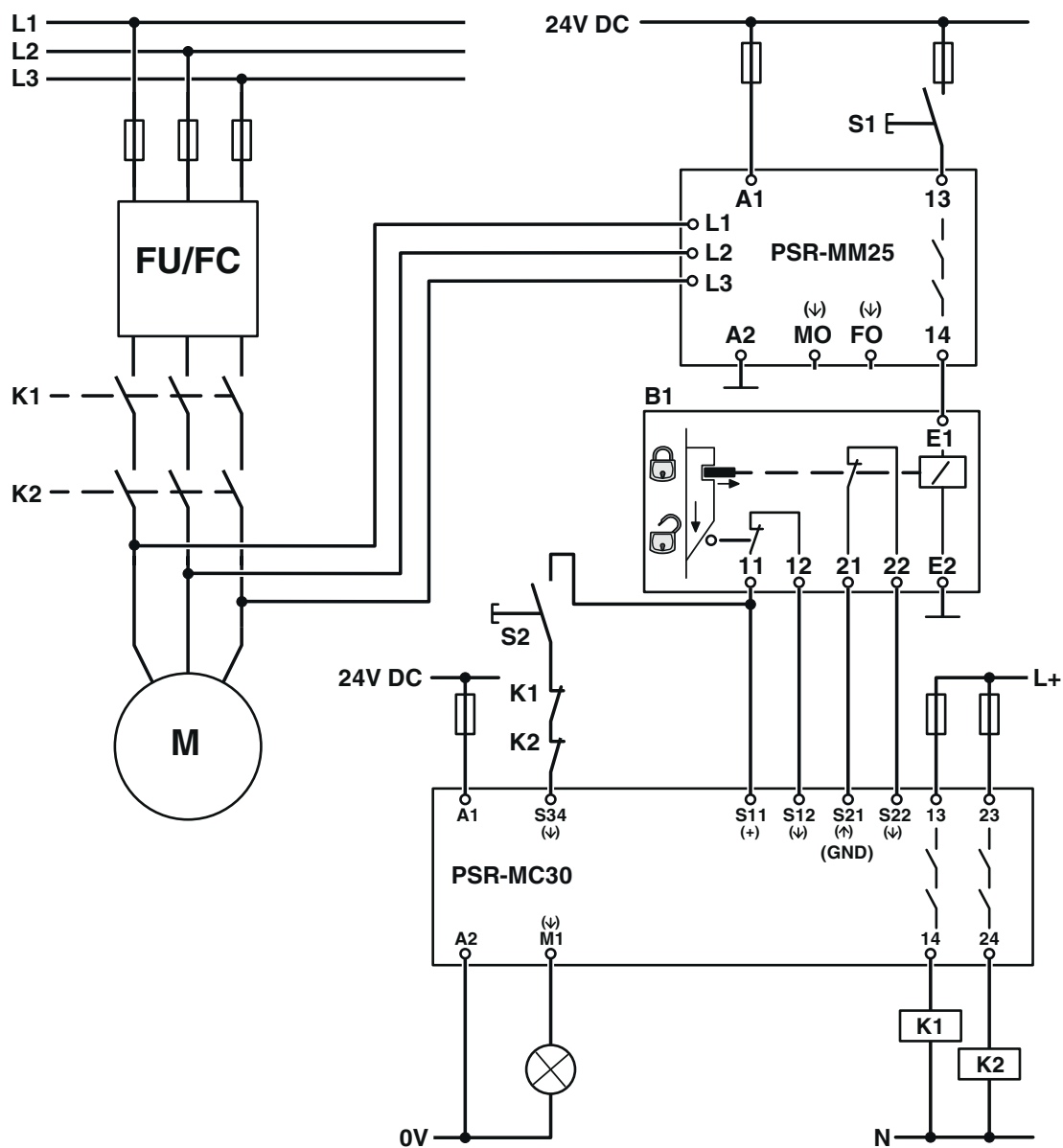
Schemat
