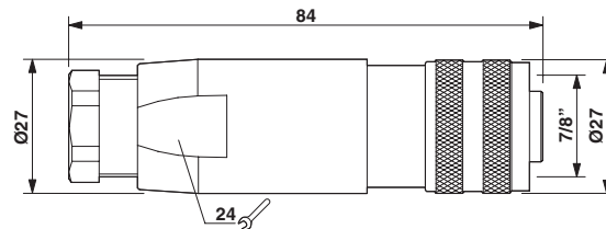
Rysunek wymiarowy
